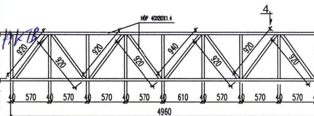
MẶT CẮT CHI TIẾT KHUNG TRÊN, DƯỚI
