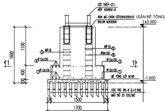
MẶT CẮT CHI TIẾT MÓNG CỘT
