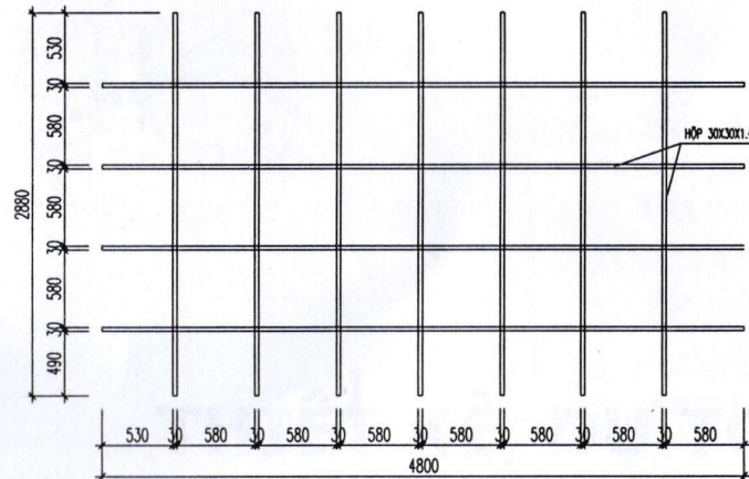
CHI TIẾT KHUNG ALUMEX SAU
