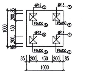
MẶT CẮT 1 - 1 MÓNG CỘT
