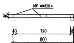
MẶT CẮT 3 - 3 CHI TIẾT KHUNG CANH
