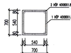
MẶT CẮT 2 - 2 KHUNG THÉP CỘT
