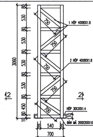
MẶT ĐỨNG KHUNG THÉP CỘT
