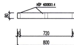
MẶT CẮT 4 - 4 CHI TIẾT KHUNG TRÊN, DƯỚI
